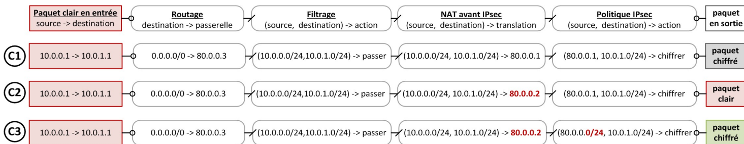
Règles de NAT avant IPsec incluses dans la politique IPsec
